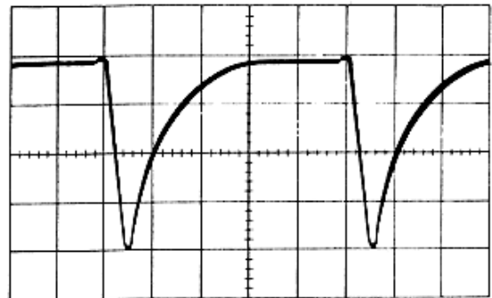
Figure 6.9 – Q14, Collector Waveform
